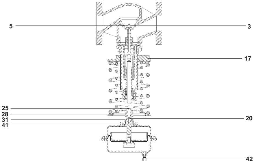
Fig. 7 - DN65 ÷ 100
