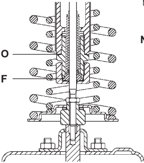
Fig. 12b - DN25 (1")
