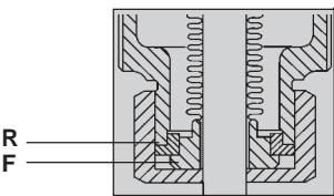
DRV4 DN65 ÷ 100
