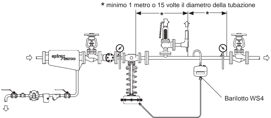
Fig. 5 - Installazione tipica per temperature a valle superiori a 125°C (90°C per diaframma in Nitrile)
