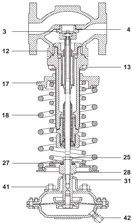
Fig. 11 - DN25 (1")
