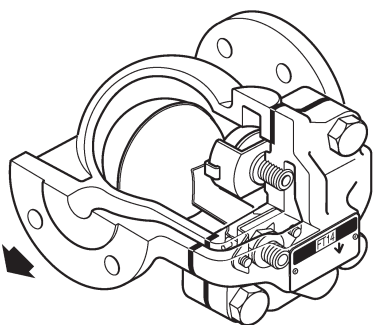
Fig. 3 FT14 (R-L) con attacchi flangiati
