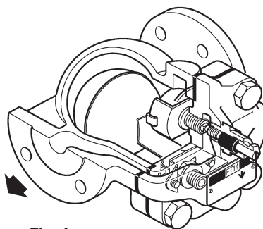
Fig. 4 FT14-C (R-L) con attacchi flangiati
