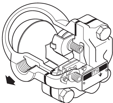
Fig. 1 FT14 (R-L) con attacchi filettati
