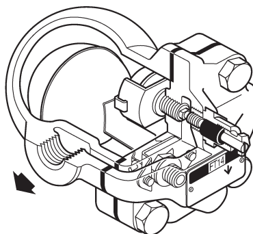
Fig. 2 FT14-C (R-L) con attacchi filettati
